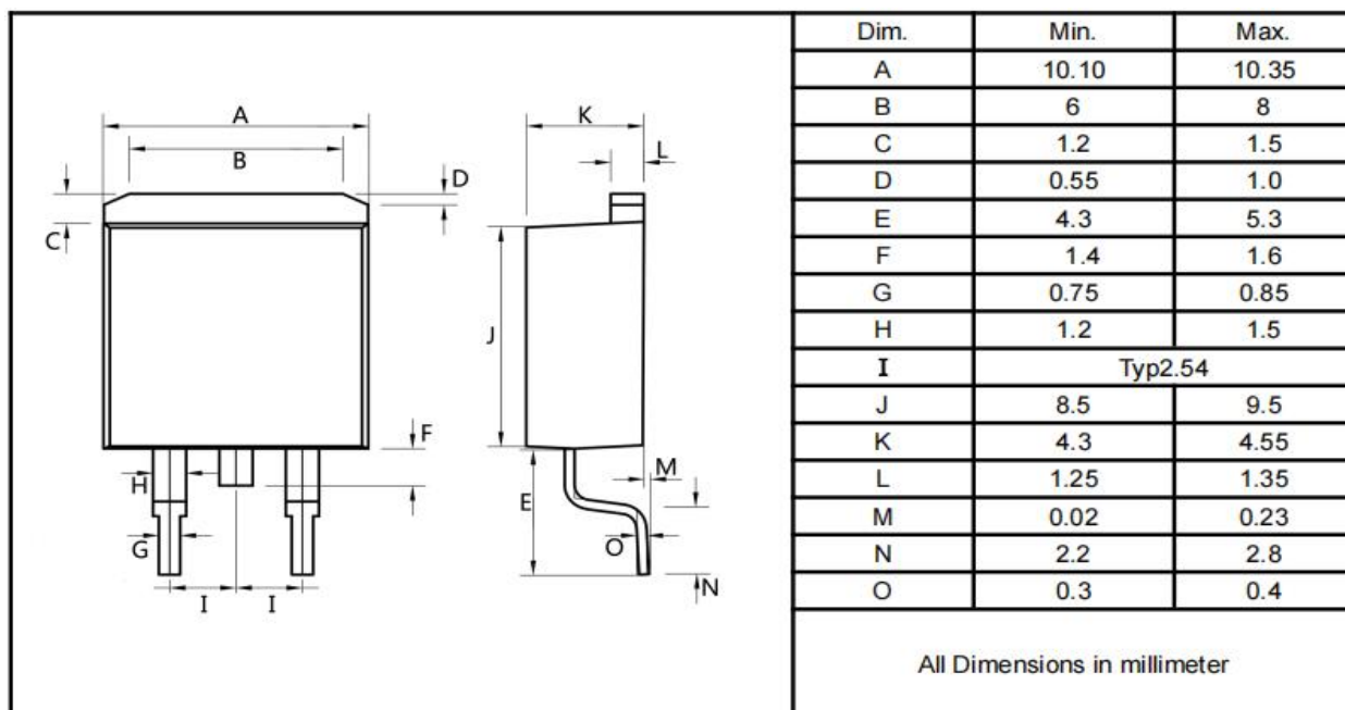
TO-263
